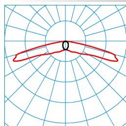
E-Line Fi L-ALB 24V Inotec L37 01 (150) TX125332
