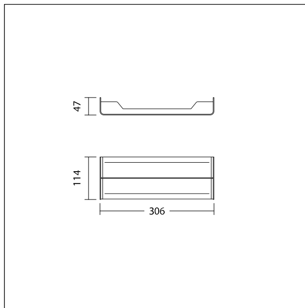
TE_ROXY_M_COUPLING.wmf
