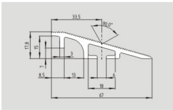
Maßzeichnung (Sonstige)
