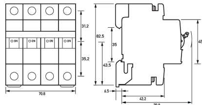
Maßzeichnung Gruppenansicht
