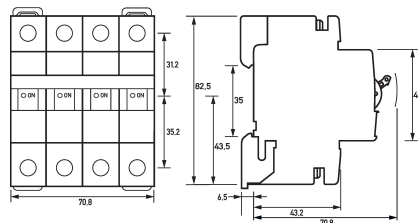
Maßzeichnung Gruppenansicht
