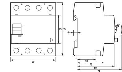
Maßzeichnung Gruppenansicht
