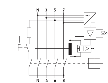
Anschlussschema
