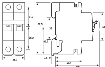
Maßzeichnung Gruppenansicht
