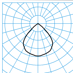
InperiaL G2 C07 BR22 2700-840 03 ■ C0 - C180 TX373344
