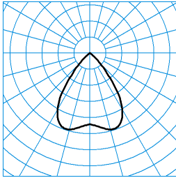
InperiaL G2 C07 BR19 1000-840 01 ■ C0 - C180 TX052562
