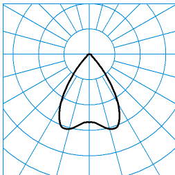
InperiaL G2 C07 BR19 1000-840 01 + ZN-PC ■ C0 - C180 TX052567
