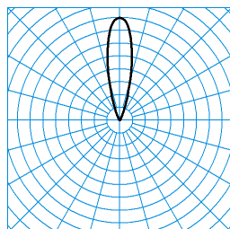
Altigo G2 90 RM3L/3000-830 1G1P + G2 VE IP66 24V DC 240W ■ C0 - C180 TX113705 DIN 5040: E04 UTE: 0,00 J + 1,00 T CEN Flux Code: 0 0 0 0 100 97 99 100 100
