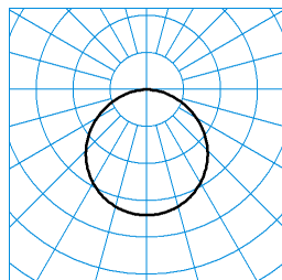
Skeo Circ MultiLC WD2 1G1Y ET (nw) ■ C0 - C180 TX278666 UGR I = 22,8 UGR q = 22,8 DIN 5040: A40 UTE: 1,00 E CEN Flux Code: 46 78 96 100 100
