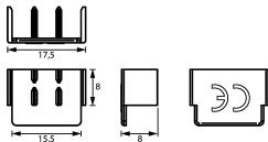
Maßzeichnung Gruppenansicht
