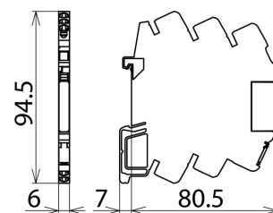
Maßbild DCO SD2 E 24
