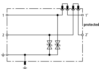
Prinzipialschaltbild DCO SD2 E 24
