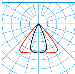
E-Line Fi Grado 50-840 J23 L37 03 (150) TX372620 ■ C0 - C180
