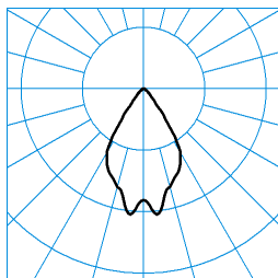
InperlaLP C05 BR19 1000-840 03 + RD-PC TX041501 ■ C0 - C180 UGR I = 16,1 UGR q = 16,1 DIN 5040: A70 UTE: 1,00 A CEN Flux Code: 88 97 99 100 100
