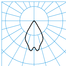
InperlaLP C05 BR19 1000-840 03 + ZN-PC TX041503 ■ C0 - C180 UGR I = 17,8 UGR q = 17,8 DIN 5040: A60 UTE: 1,00 A CEN Flux Code: 87 95 98 99 100 33 56 67 1
