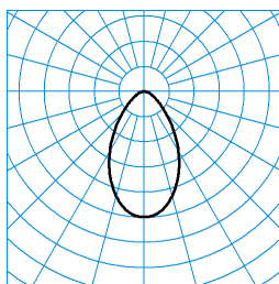
InperlaLP C05 BR19 1000-840 03 + DA-M 03 TX041500 ■ C0 - C180 UGR I = 22,9 UGR q = 22,9 DIN 5040: A50 UTE: 1,00 B CEN Flux Code: 71 91 98 100 100
