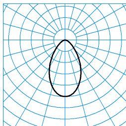
InperlaLP C05 BR19 1000-840 03 + DA-M 01 TX041499 ■ C0 - C180 UGR I = 22,9 UGR q = 22,9 DIN 5040: A50 UTE: 1,00 B CEN Flux Code: 71 91 98 100 100
