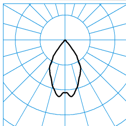
InperlaLP C05 BR19 1000-840 03 TX040938 ■ C0 - C180 UGR I = 16,7 UGR q = 16,7 DIN 5040: A70 UTE: 1,00 A CEN Flux Code: 96 100 100 100 100
