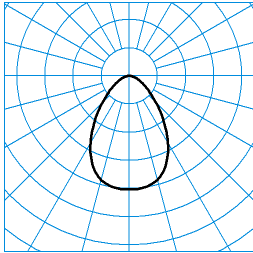
InperiaL G2 C07 BR25 4700-830 03 + DA-M 03 ■ C0 - C180 TX373531
