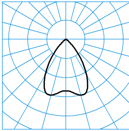
InperiaL G2 C07 BR25 4700-830 03 + RD-PC ■ C0 - C180 TX373530
