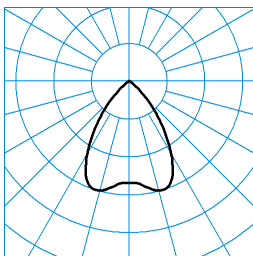
InperiaL G2 C07 BR25 4700-830 03 + DA 03 ■ C0 - C180 TX373532
