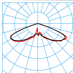
Publisca P1-RB6L-LR/2000-740 3G1S TX047629
