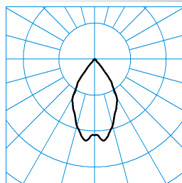
InperlaLP C05 BR19 1000-830 03 TX369702 ■ C0 - C180
