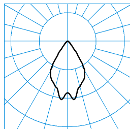
InperlaLP C05 BR19 1000-830 03 + RD-PC TX369707 ■ C0 - C180
