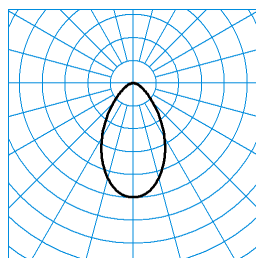
InperlaLP C05 BR19 1000-830 03 + DA-M 03 TX369706 ■ C0 - C180
