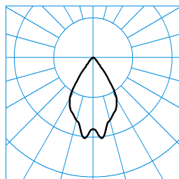
InperlaLP C05 BR19 1000-830 03 + RG-PC ■ C0 - C180 TX369708
