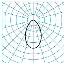
InperlaLP C05 BR19 1000-830 03 + DA-M 01 TX369705 ■ C0 - C180
