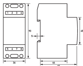
Maßzeichnung Gruppenansicht
