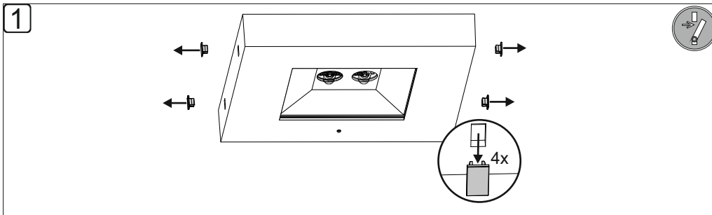
Demontage der Abdeckung: / demounting of covering
