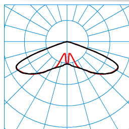
Publisca P1-RB6L-LR/1100-730 2G1S TX047616
