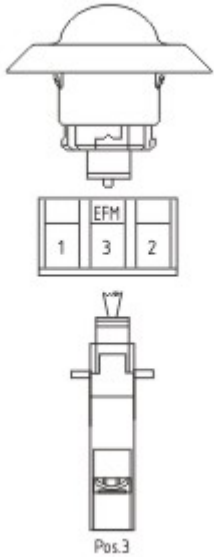
Anwendungsbeispiel
