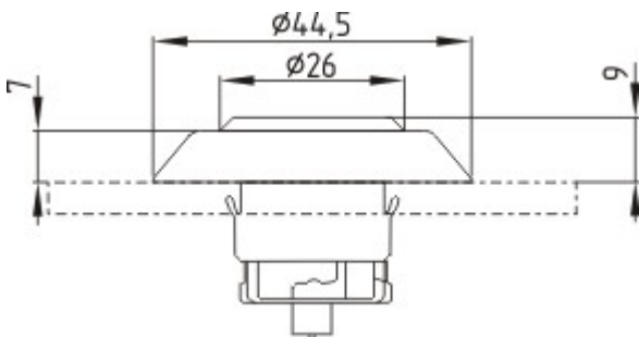
Maßzeichnung (Grundgerät)
