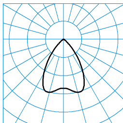
InperiaL G2 C07 HR19 2700-830 01 + RD-PC ■ C0 - C180 TX372388
