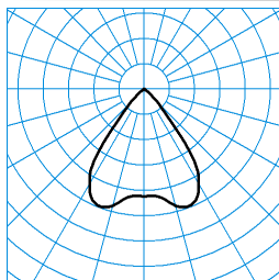
InperiaL G2 C07 HR19 2700-830 01 ■ C0 - C180 TX372384
