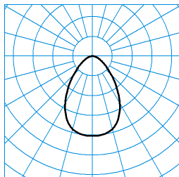
InperiaL G2 C07 HR19 2700-830 01 + DA-M 01 ■ C0 - C180 TX372387
