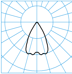
InperlaLP C05 HR22 2700-830 03 + RD-PC ■ C0 - C180 TX041723
