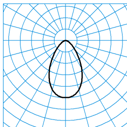
InperlaLP C05 HR22 2700-830 03 + DA-M 03 TX041722 ■ C0 - C180
