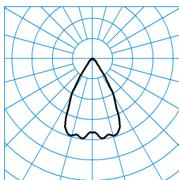
InperlaLP C05 HR22 2700-830 03 + RG-PC TX041724 ■ C0 - C180
