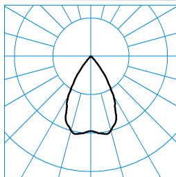
InperlaLP C05 HR22 2700-830 03 TX040976 ■ C0 - C180
