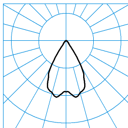
InperlaLP C05 HR22 2700-830 03 + ZN-PC TX041725 ■ C0 - C180
