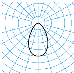
InperlaLP C05 HR22 2700-830 03 + DA-M 01 TX041721 ■ C0 - C180
