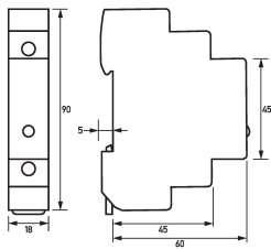
Maßzeichnung Gruppenansicht
