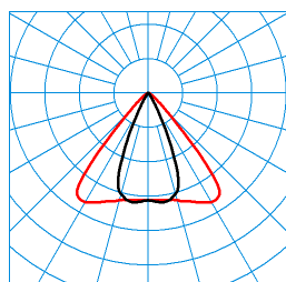
E-Line Fi Grado 50-840 J23 L37 05 (225) TX123812 ■ C0 - C180
