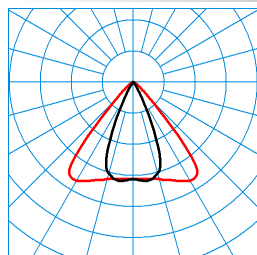
E-Line Fi Grado 40-840 J23 L37 05 (225) TX123815 ■ C0 - C180
