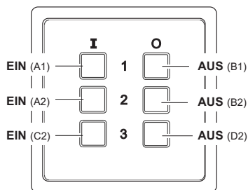
RTS14E5003-01 EIN/AUS 2-Tast-Bedienung
