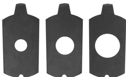
Im Lieferumfang enthaltene Fixkonturen (Kreise – siehe Abb. 1) Included fixed contours (circles – see fig. 1)
