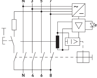
Anschlusschema
