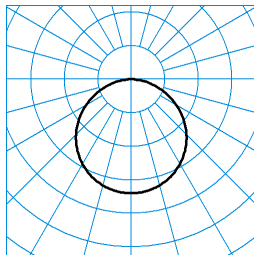
Skeo Circ MultiLC WD2 1G1Y ET E3 (ww) ■ C0 - C180 TX374646 UGR I = 22,8 UGR q = 22,8 DIN 5040: A40 UTE: 1,00 E CEN Flux Code: 46 78 96 100 100
