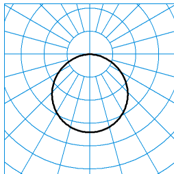
Skeo Circ MultiLC WD2 1G1Y ET E3 (nw) ■ C0 - C180 TX278649 UGR I = 22,8 UGR q = 22,8 DIN 5040: A40 UTE: 1,00 E CEN Flux Code: 46 78 96 100 100
