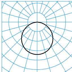
Skeo Circ MultiLC WD2 1G1Y ET E3 (cw) ■ C0 - C180 TX278635 UGR I = 22,8 UGR q = 22,8 DIN 5040: A40 UTE: 1,00 E CEN Flux Code: 46 78 96 100 100
