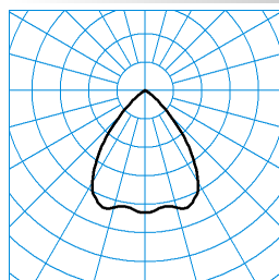
InperiaLP C05 BR22 1000-830 03 TX374006 ■ C0 - C180
