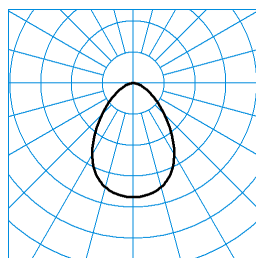
InperiaLP C05 BR22 1000-830 03 + DA-M 01 TX374001 ■ C0 - C180
