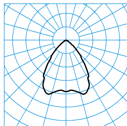
InperiaLP C05 BR22 1000-830 03 + RD-PC TX373114 ■ C0 - C180
