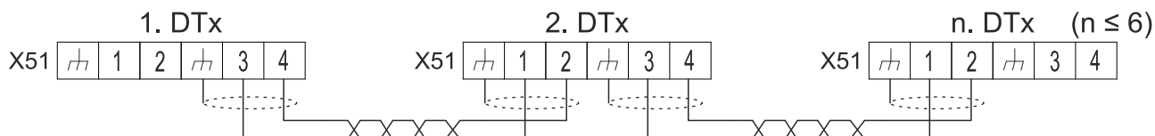
Рис. 11: Мультимастерное управление
