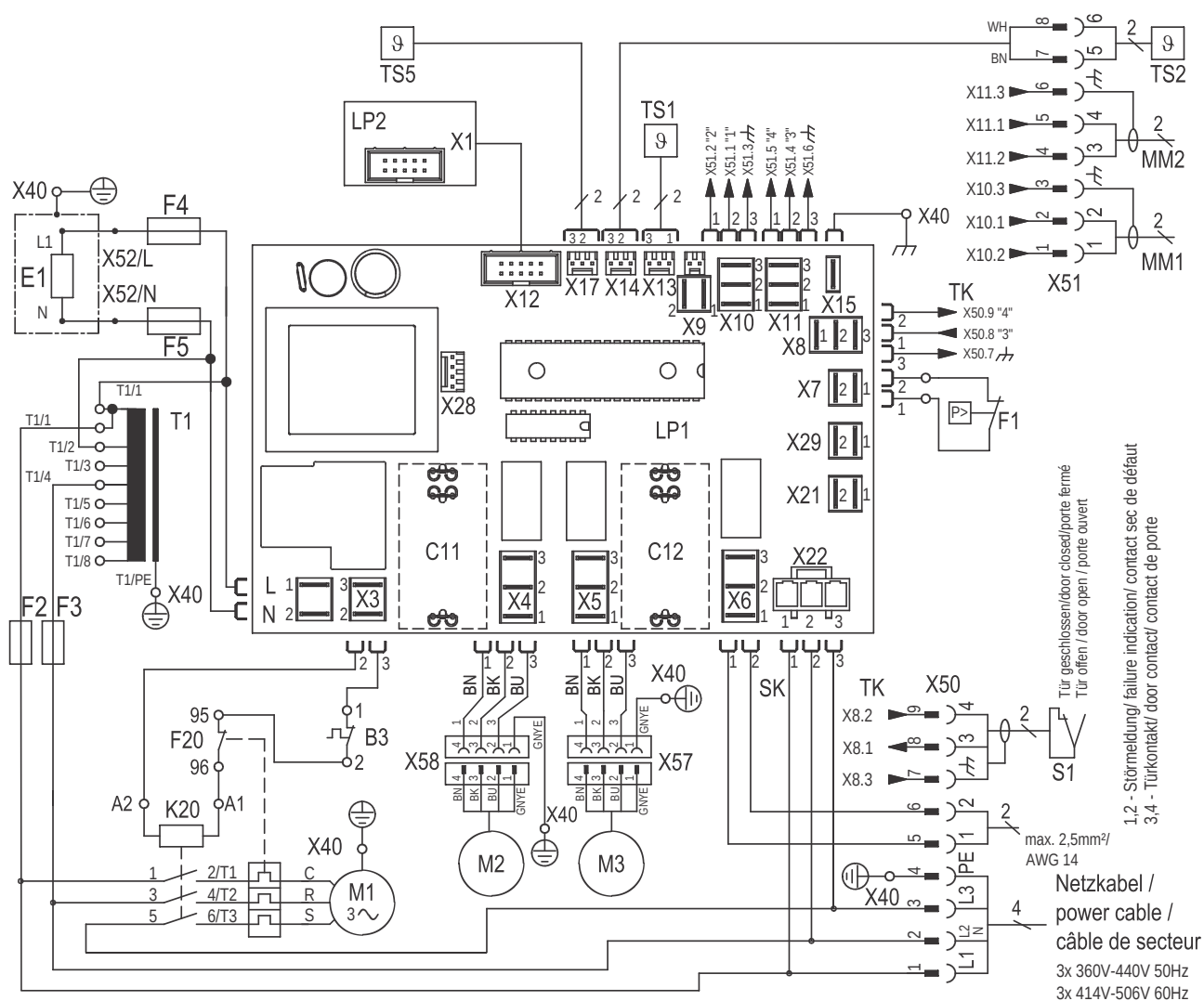
Abb. 21: Stromlaufplan
