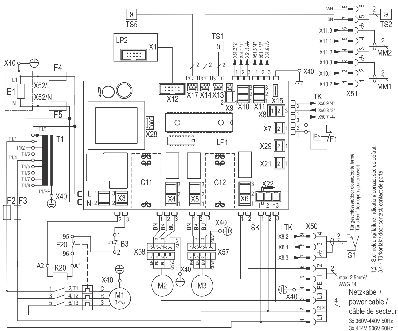
Fig. 21: Esquema eléctrico
