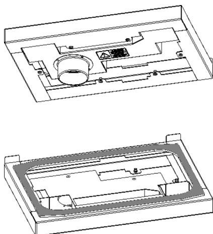
Рис. 5.: PAD-рама
