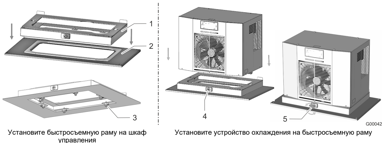
Рис. 20: Монтаж держателя
