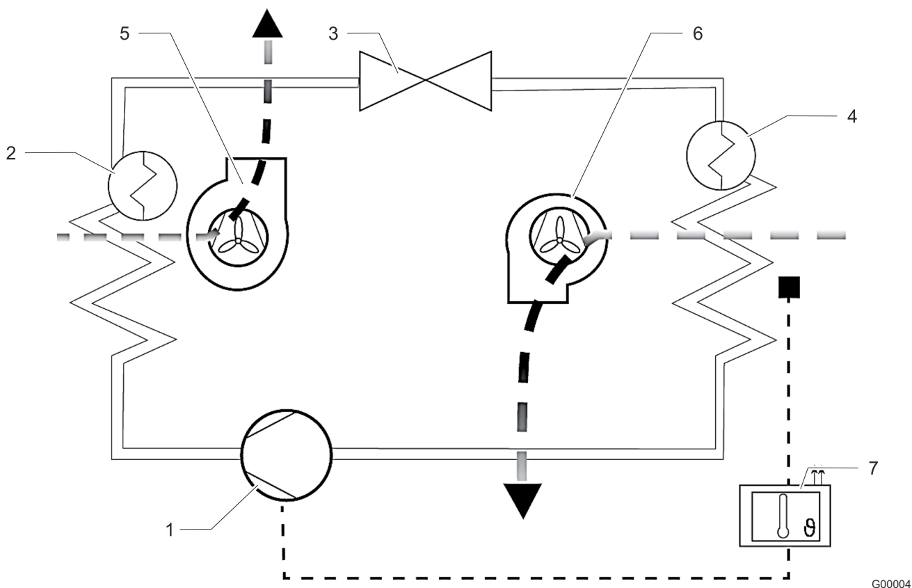
Рис. 7.: Холодильный контур
