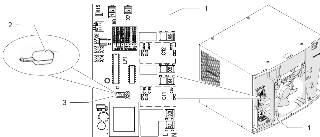
Abb. 28: Serviceschnittstelle
