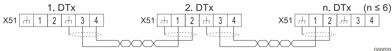
Fig. 11 : Commande multimaître
