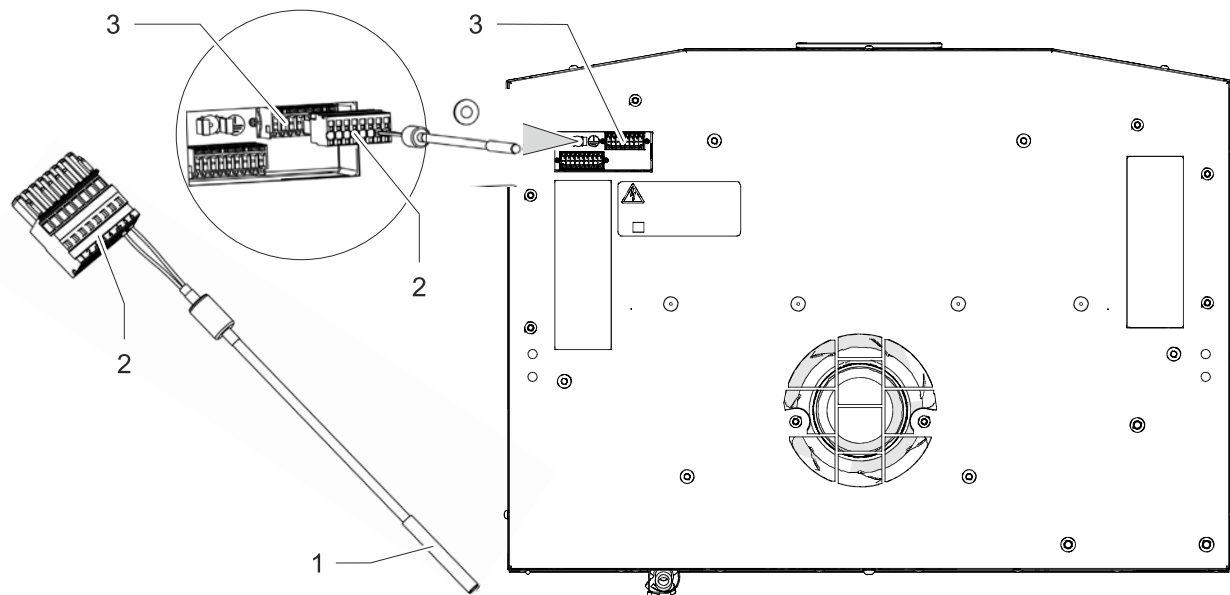
Abb. 10: Temperatursensor - TS2
