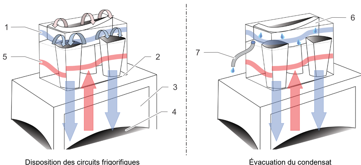
Disposition des circuits frigorifiques Fig. 8 : circuits frigorifiques et évacuation du condensat
