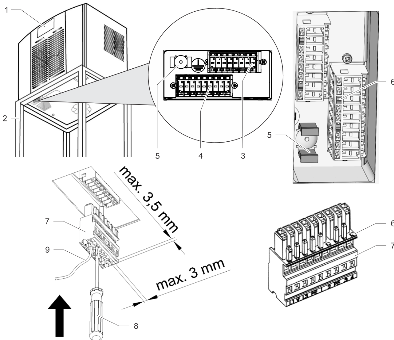
Fig. 24 : fiche de raccordement secteur du climatiseur
