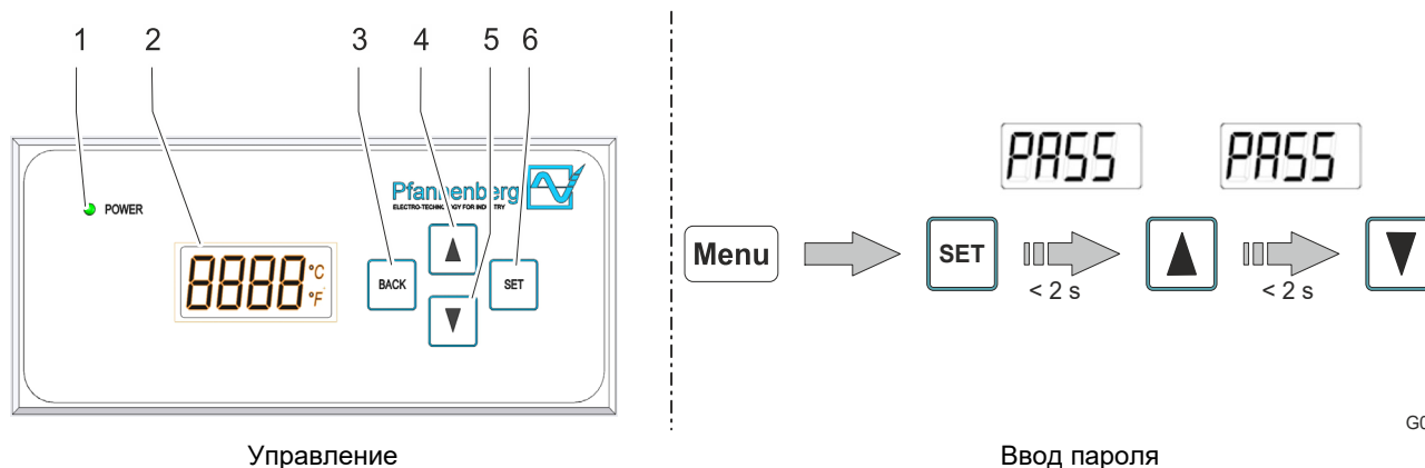
Рис. 27.: Блок управления мультиконтроллера (MC)
