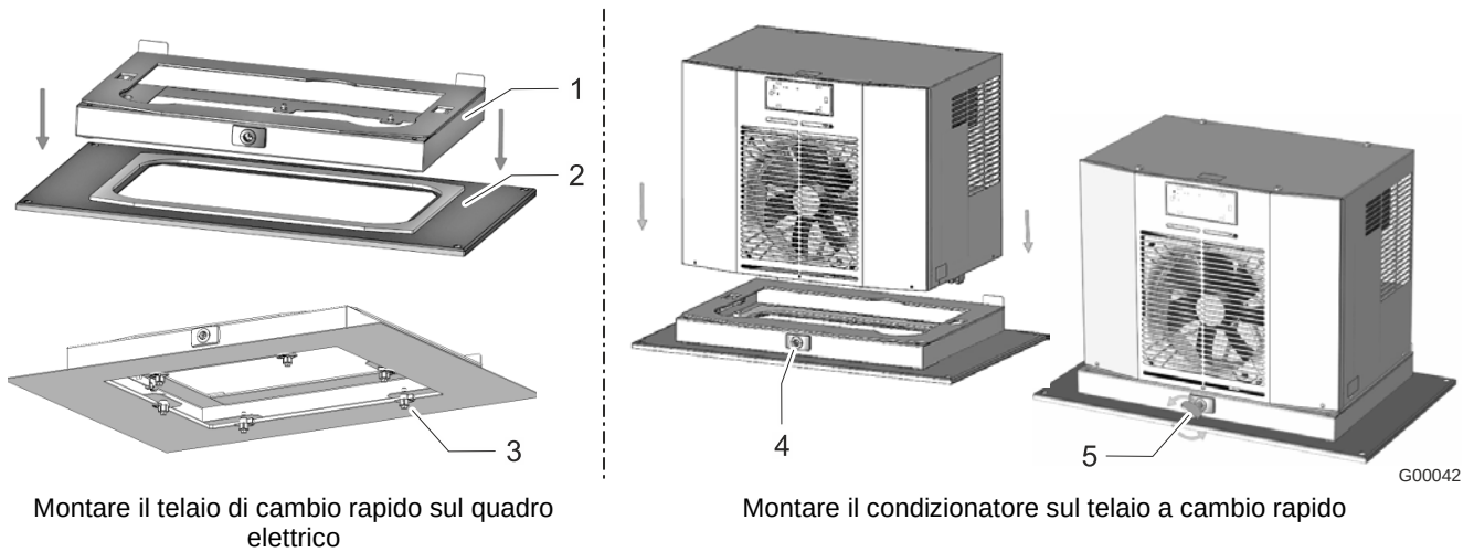
Fig. 20: Montare la staffa
