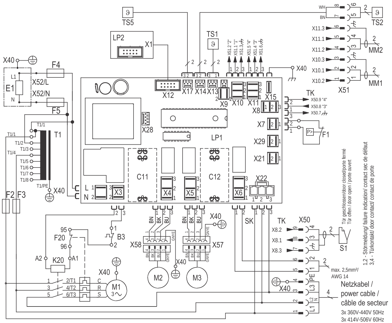
Fig. 21: Schema elettrico
