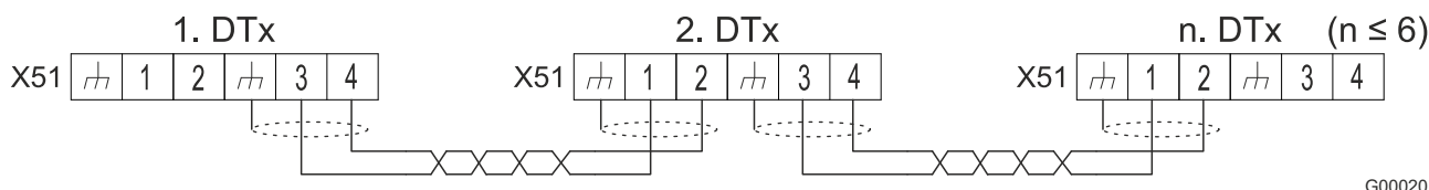
Fig. 22: Commande multimaître
