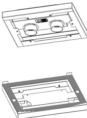
PAD-рама (двухканальная система*) Устройства охлаждения DTT 6301/6401
