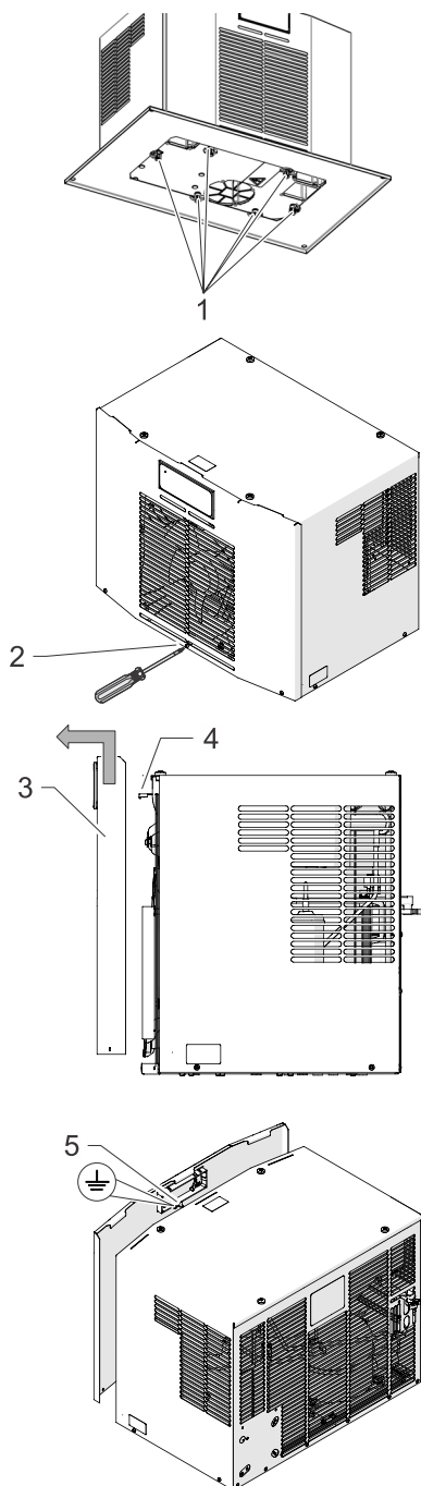
Fig. 17: Retirada de la tapa frontal
