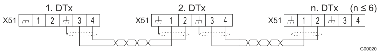
Рис. 22.: Мультимастерное управление
