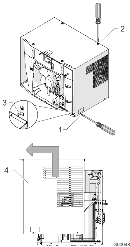
Abb. 18: Gerätehaube entfernen
