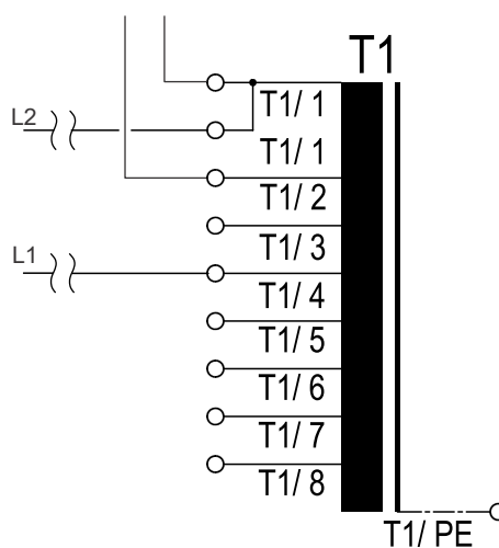
Devanado de entrada del transformador de control
