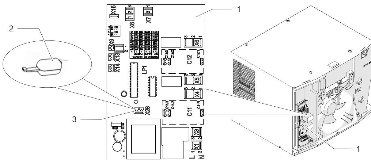
Рис. 28: Сервисный интерфейс
