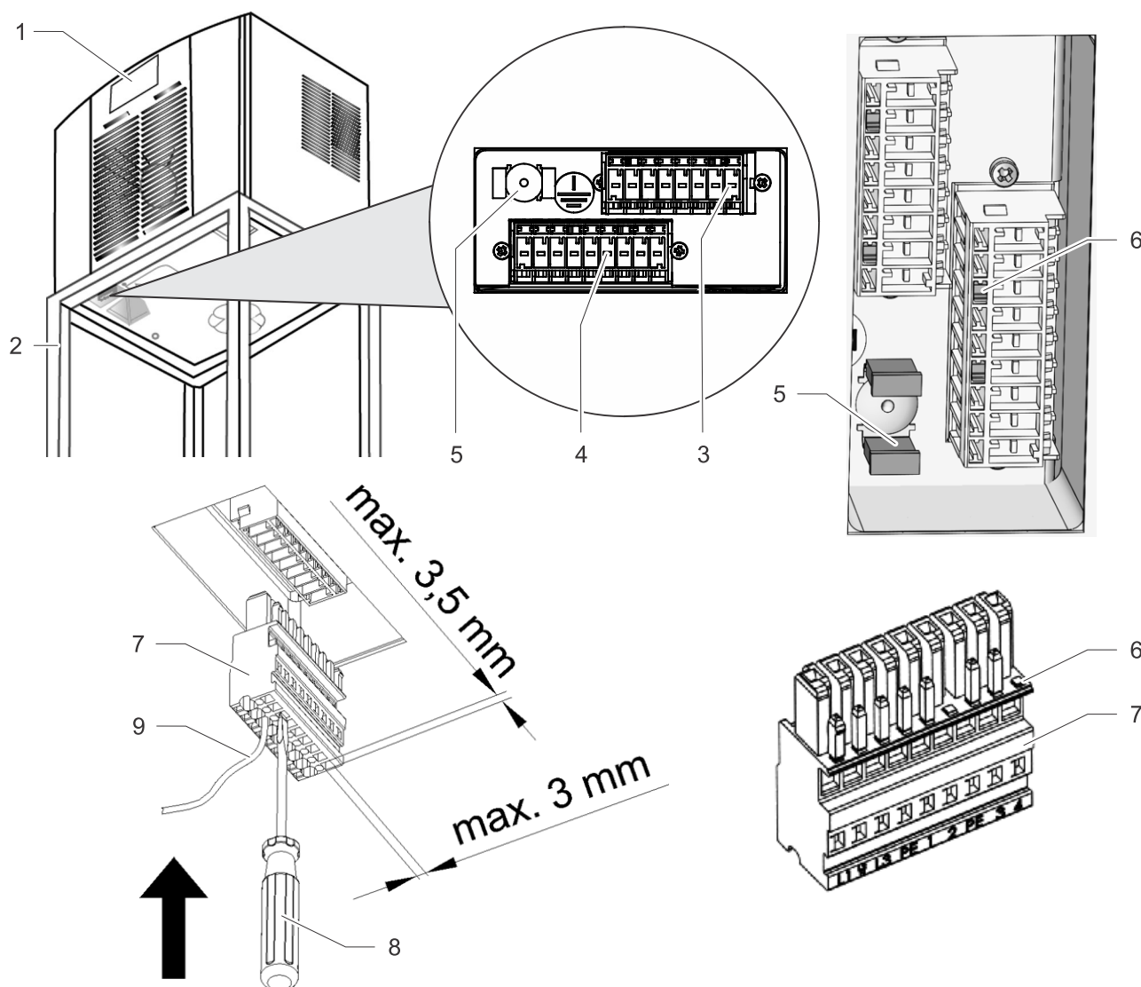
Рис. 24: Сетевой разъем устройства охлаждения
