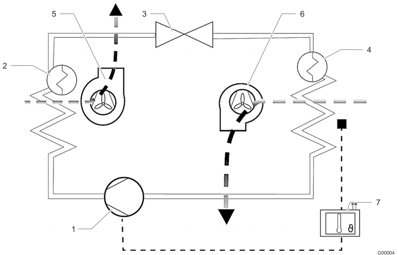
Abb. 7: Kältekreislauf
