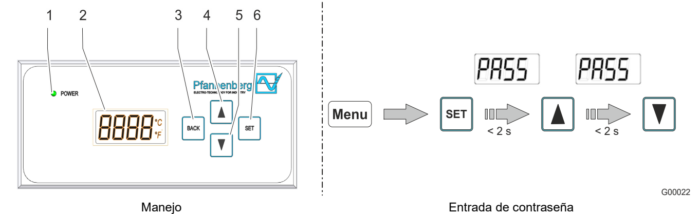
Fig. 27: Manejo del multicontrolador (MC)
