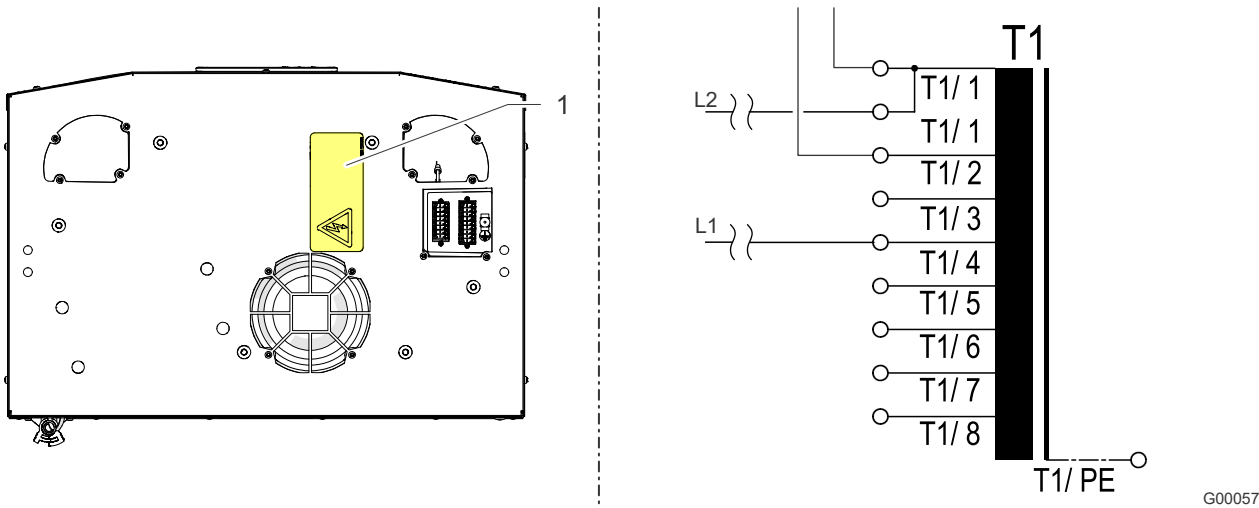
Заводские настройки управляющего трансформатора Входная обмотка управляющего трансформатора Рис. 25: Настройка сетевого напряжения на управляющем трансформаторе
