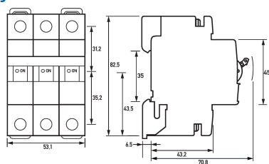
Maßzeichnung Gruppenansicht
