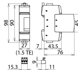
Maßbild DG SE CI WE 440 FM
