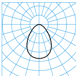
InperiaLP C05 BR22 1800-840 03 + DA-M 03 TX041552
