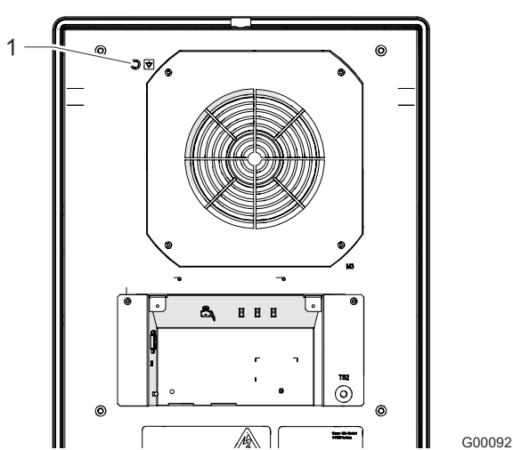
Fig. 21: Equipotential bonding
