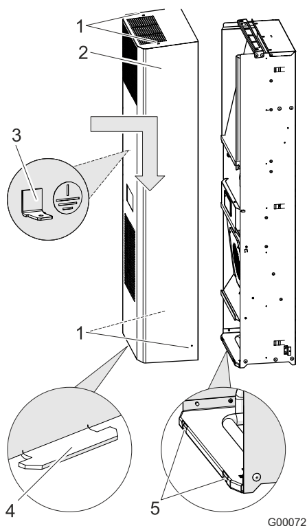
Fig. 26 : montage du capot de l'appareil
