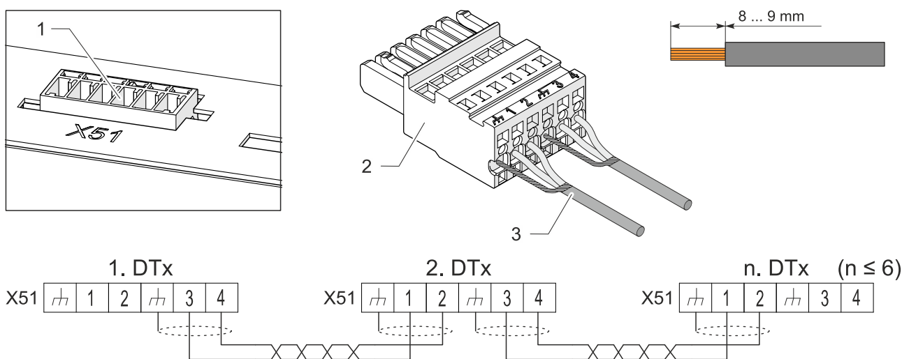
Fig. 17: commande multimaître
