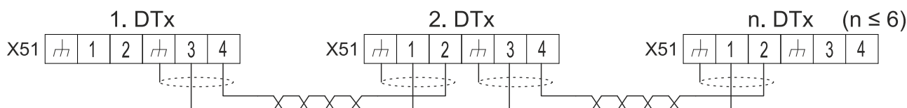
Рис. 8: Мультимастерное управление
