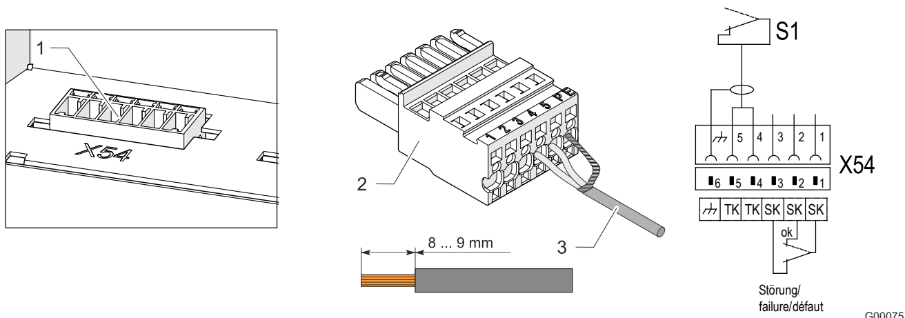
Fig. 18: Conexión del interruptor de contacto de puerta
