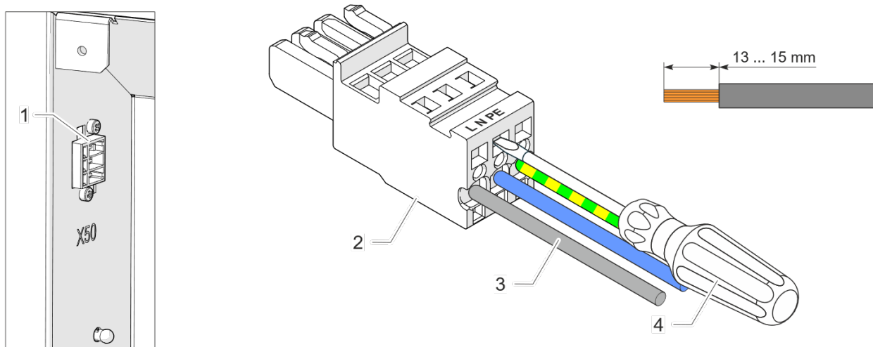
Fig. 20: Connettore di collegamento alla rete del condizionatore
