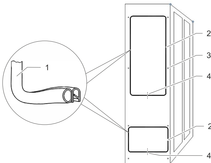
Fig. 12: Colocación del sellado del perfil
