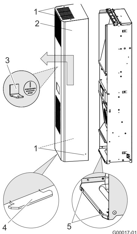
Fig. 25: Desmontaje del protector de la unidad
