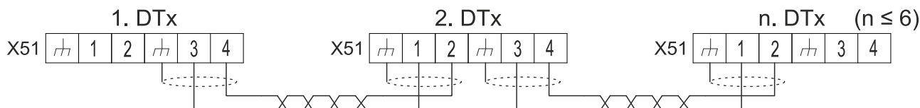
Fig. 8 : commande multimaître
