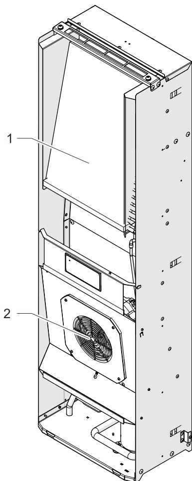
Abb. 27: Wärmetauscher reinigen
