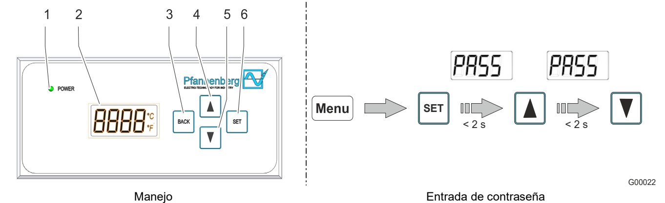
Fig. 23: Manejo del multicontrolador (MC)
