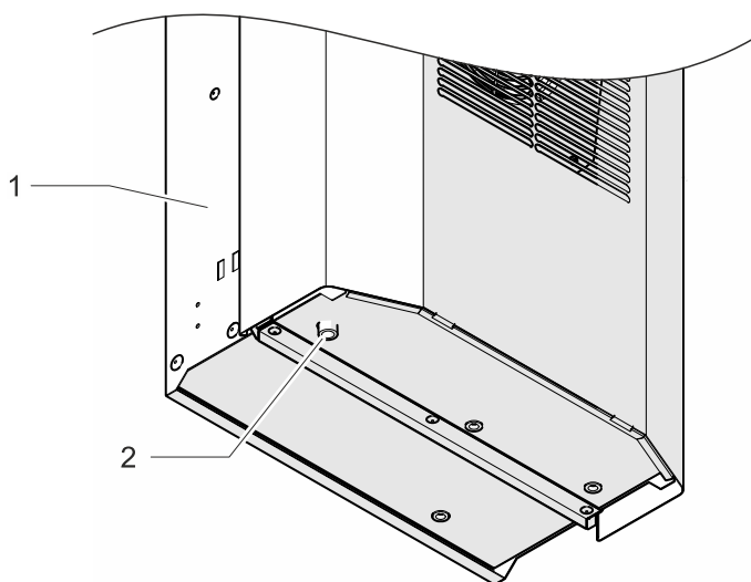
Рис. 6: Сливной патрубок конденсата (пример: устройство охлаждения DTI)
