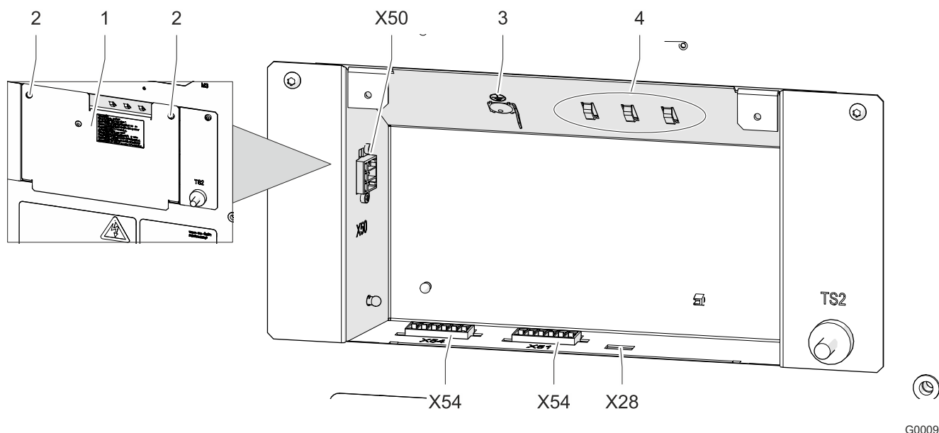
Fig. 16: Vano terminali
