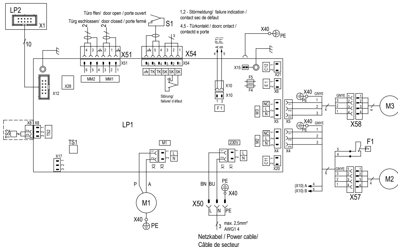
Abb. 15: Stromlaufplan
