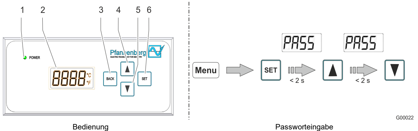
Abb. 23: Bedienung Multi-Controller (MC)
