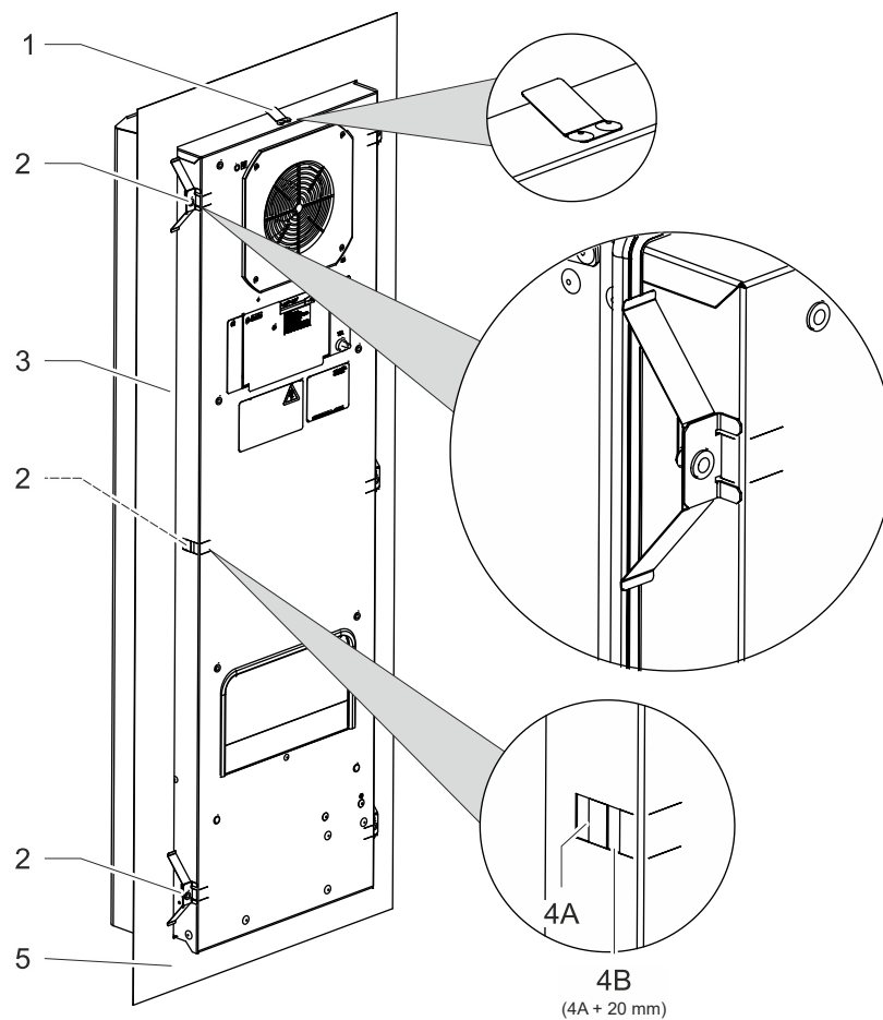
Abb. 14: Kühlgerät montieren
