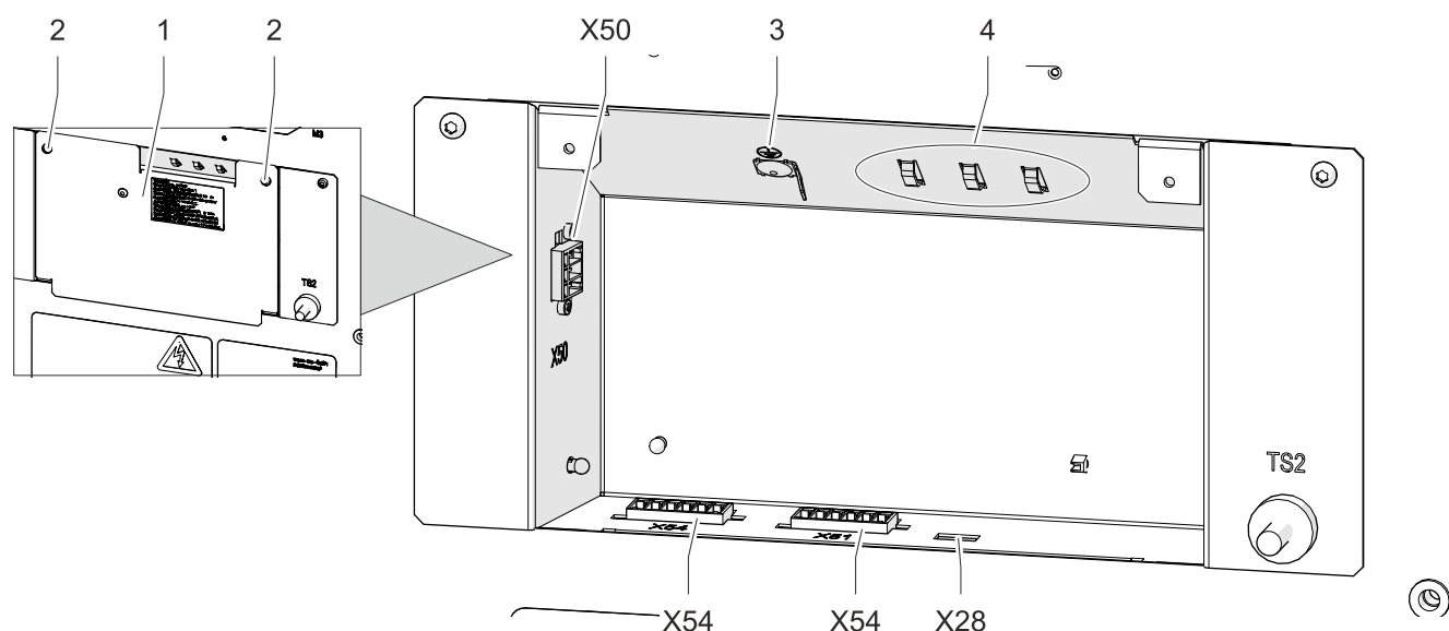
Abb. 16: Anschlussraum
