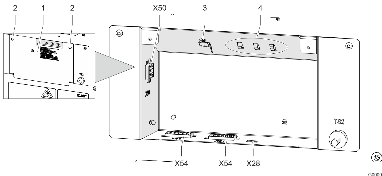
Fig. 16 : compartiment de raccordement
