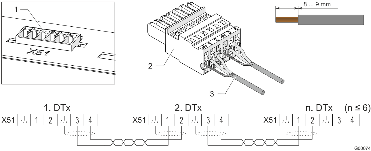
Рис. 17.: Мультимастерное управление
