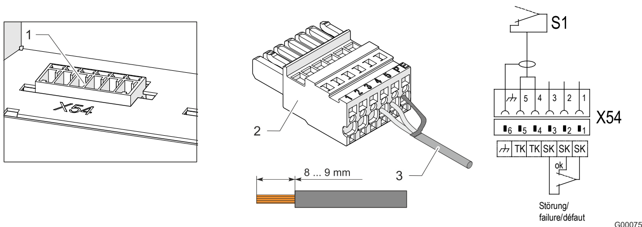
Abb. 18: Türkontaktschalter anschließen
