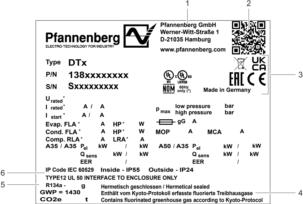
Abb. 9: Typenschild (Beispiel)
