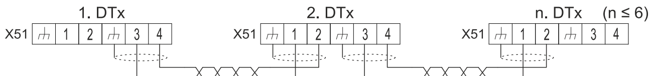
Abb. 8: Multimaster-Steuerung
