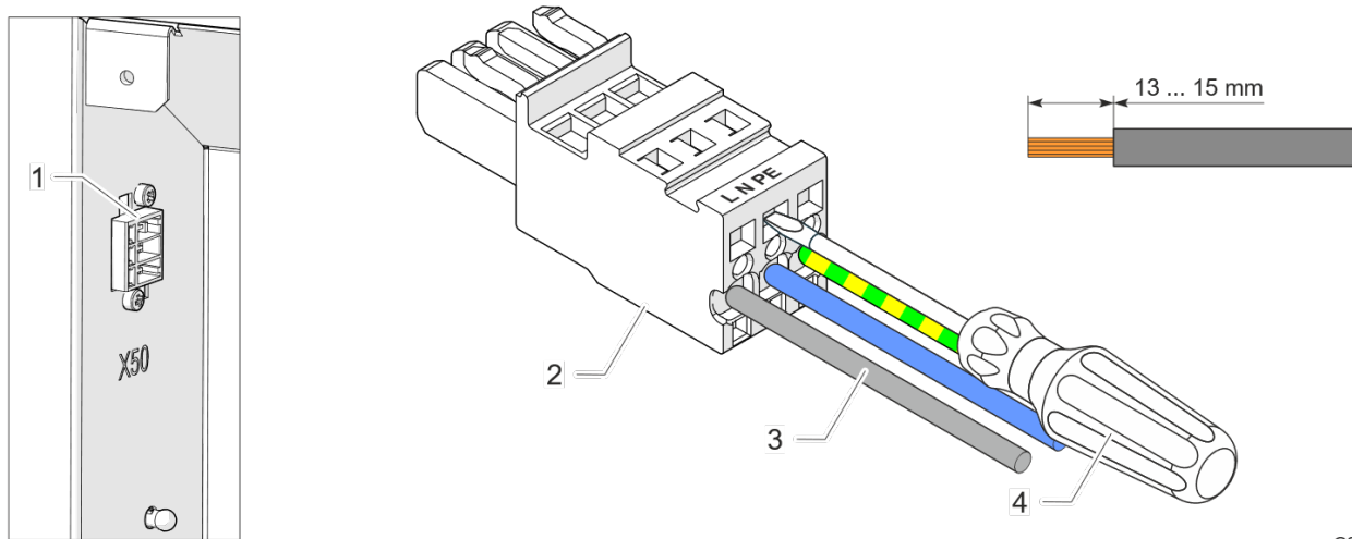
Fig. 20: Conector de conexión a la red del climatizador
