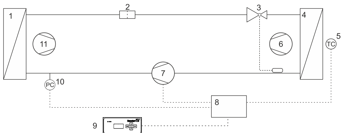
Рис. 5.: Холодильный контур
