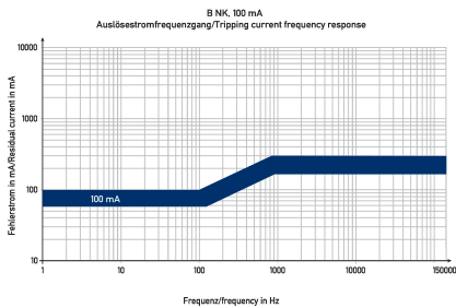
Kennlinie B NK 100 mA
