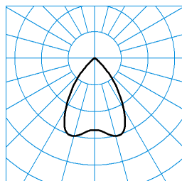
InperlaL G2 C07 HR19 1000-840 03 + RG-PC ■ C0 - C180 TX373546
