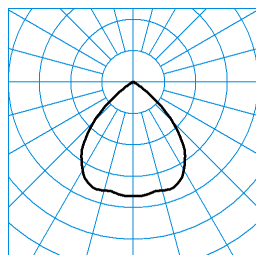
InperlaL G2 C07 HR22 2700-830 01 + RG-PC ■ C0 - C180 TX373484
