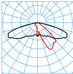
Publisca P1W-AB2L-LR/3800-740 6G1S TX053488 ■ C0 - C180 ■ C90 - C270 DIN 5040: A30 UTE: 1,00 G CEN Flux Code: 34 72 97 100 100 0 0 0 0
