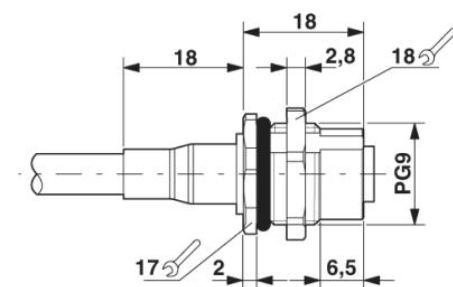
M12 Wanddurchführung
