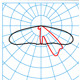
Publisca P1-AB2L-LR/2000-740 3G1S TX047518
