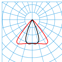
E-Line Fi Grado 30-840 J23 L37 03 (150) TX125315 ■ C0 - C180 UGR I = 26,6 UGR q = 10,6 DIN 5040: A70 UTE: 0,93 A CEN Flux Code: 92 99 100 100 93
