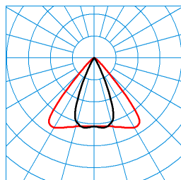
E-Line Fi Grado 30-830 J21 L37 03 (150) TX123672 ■ C0 - C180 ■ C90 - C270 UGR I = 26,4 UGR q = 10,4 DIN 5040: A70 UTE: 0,93 A CEN Flux Code: 92 99 100 100 93
