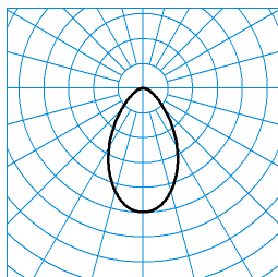
InperlaLP C05 BR19 1000-840 03 + DA-M 01 TX371113 ■ C0 - C180
