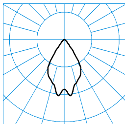
InperlaLP C05 BR19 1000-840 03 + RD-PC TX371115 ■ C0 - C180
