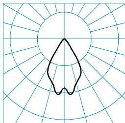
InperlaLP C05 BR19 1000-840 03 + ZN-PC TX371118 ■ C0 - C180
