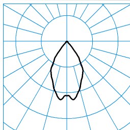
InperlaLP C05 BR19 1000-840 03 TX371098 ■ C0 - C180
