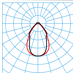
SFlow C2-L CDP-I LED4000-840 UR 01 TX133403
