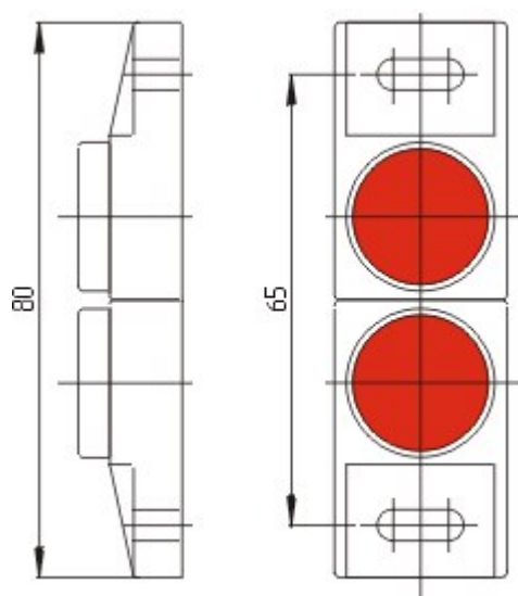
Maßzeichnung (Sonstige)
