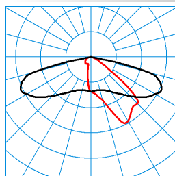
Publisca P3-AB2L-LR/1800-730 2G1 TX195593
