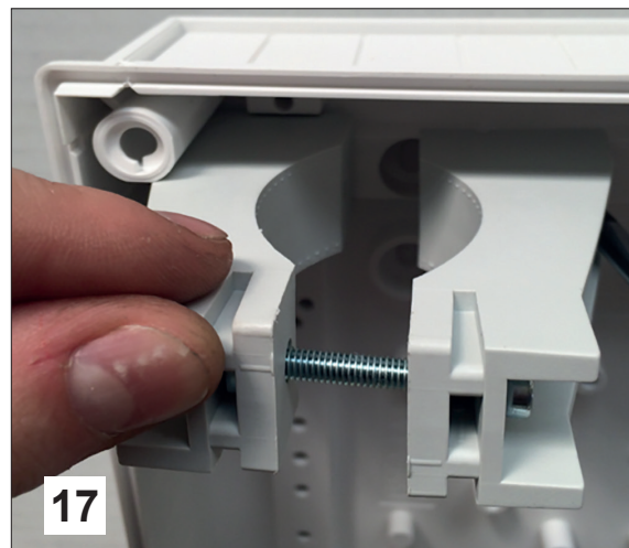
17 Kabelabfangschelle montieren
