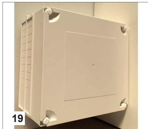
19 Einspeisegehäuse verschließen
