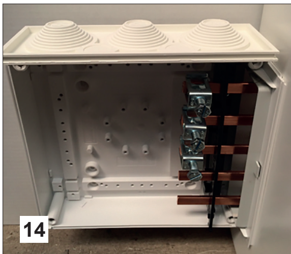
14 Einspeisegehäuse anbringen und Anordnung Einführungsflansch festlegen
