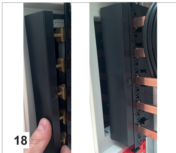
18 Sammelschienenabdeckung montieren
