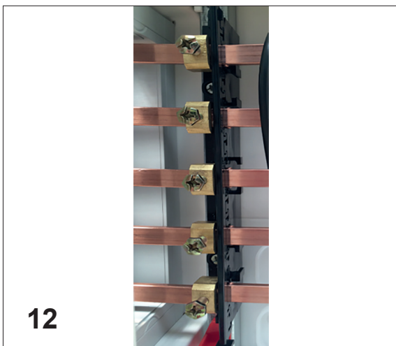
Verbindungsklemmen anbringen
