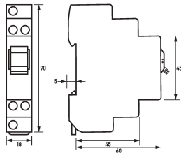
Maßzeichnung Gruppenansicht
