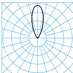
Altigo G2 30 RB17L/900-830 1G1P + G2 VE IP66 24V DC 80W ■ C0 - C180 TX113936
